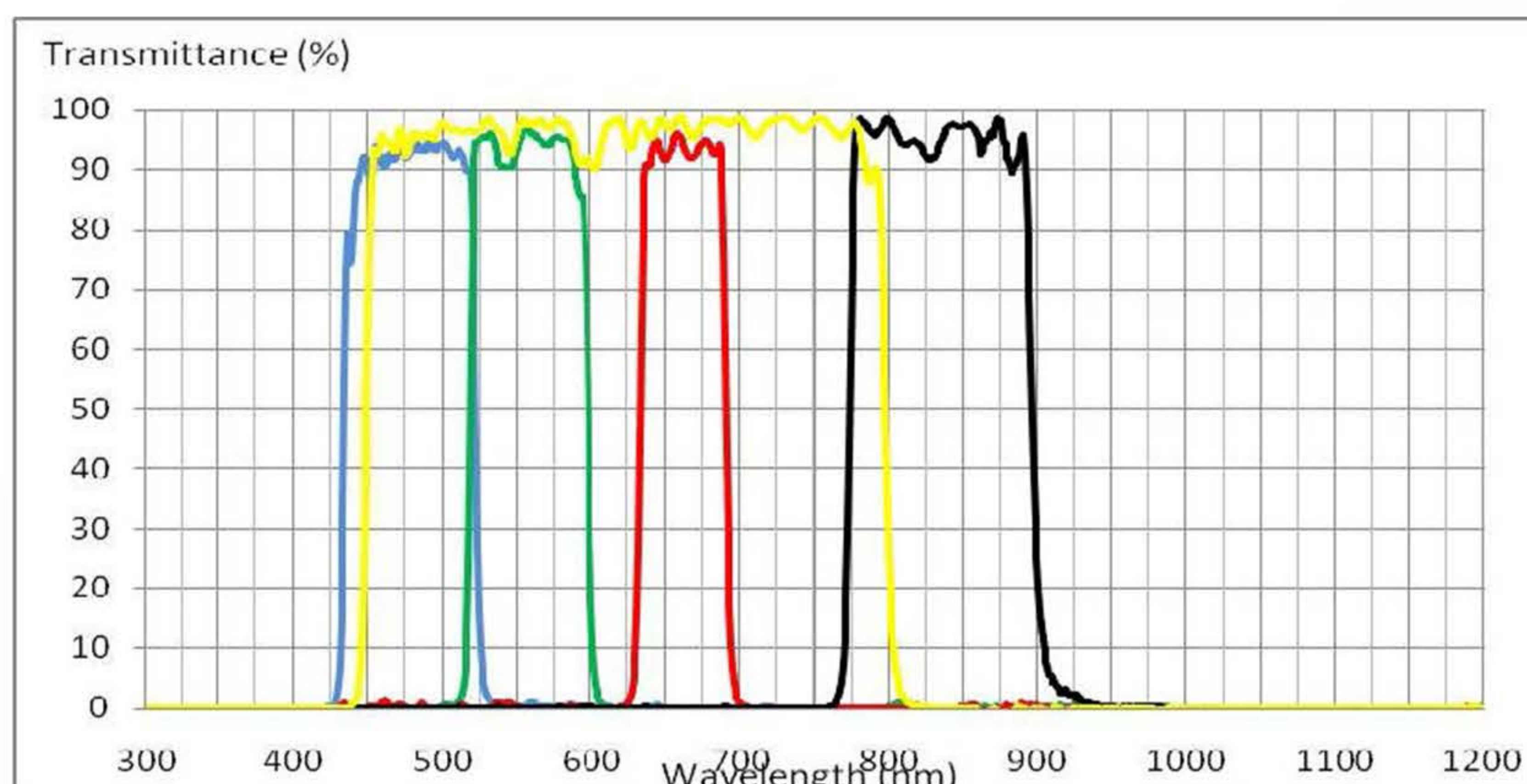
5通道多光谱滤光片光谱
