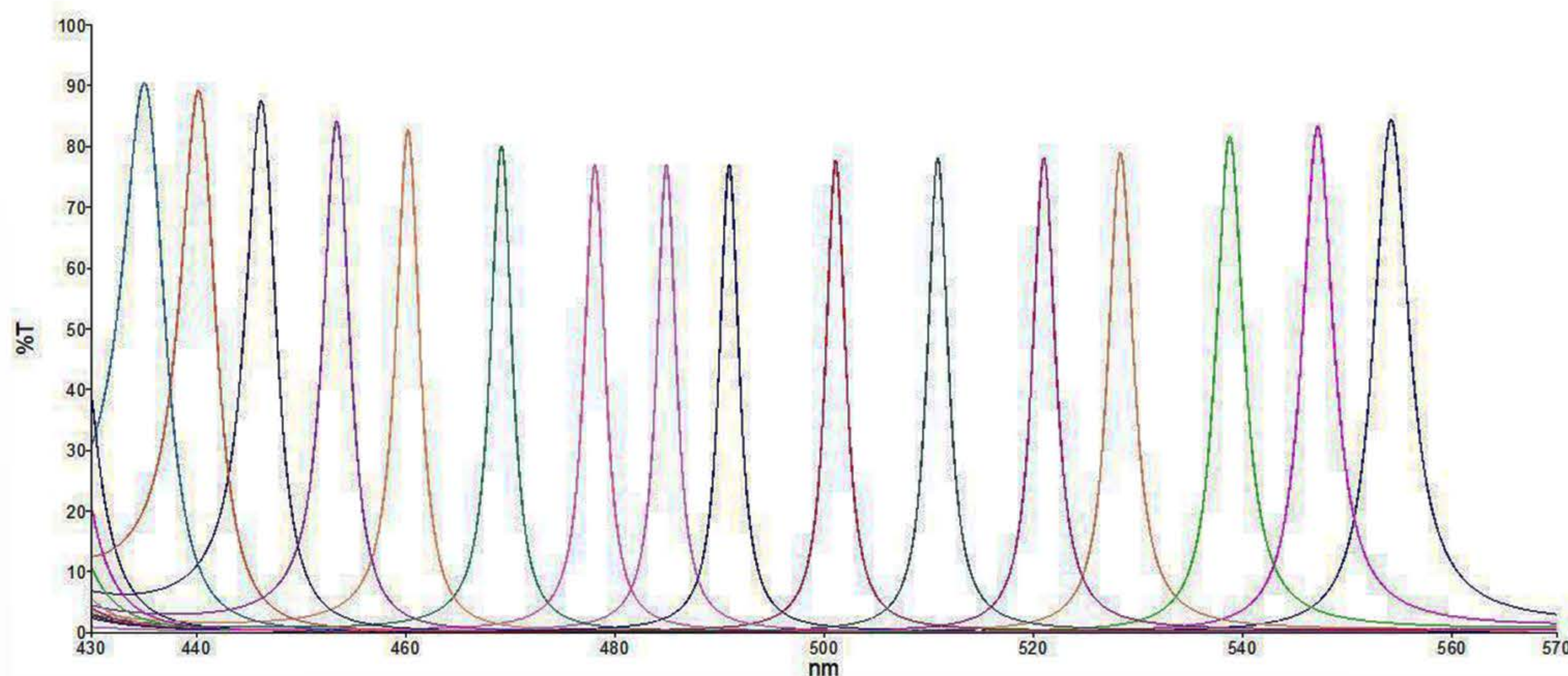
16通道420-570nm波段光谱曲线
