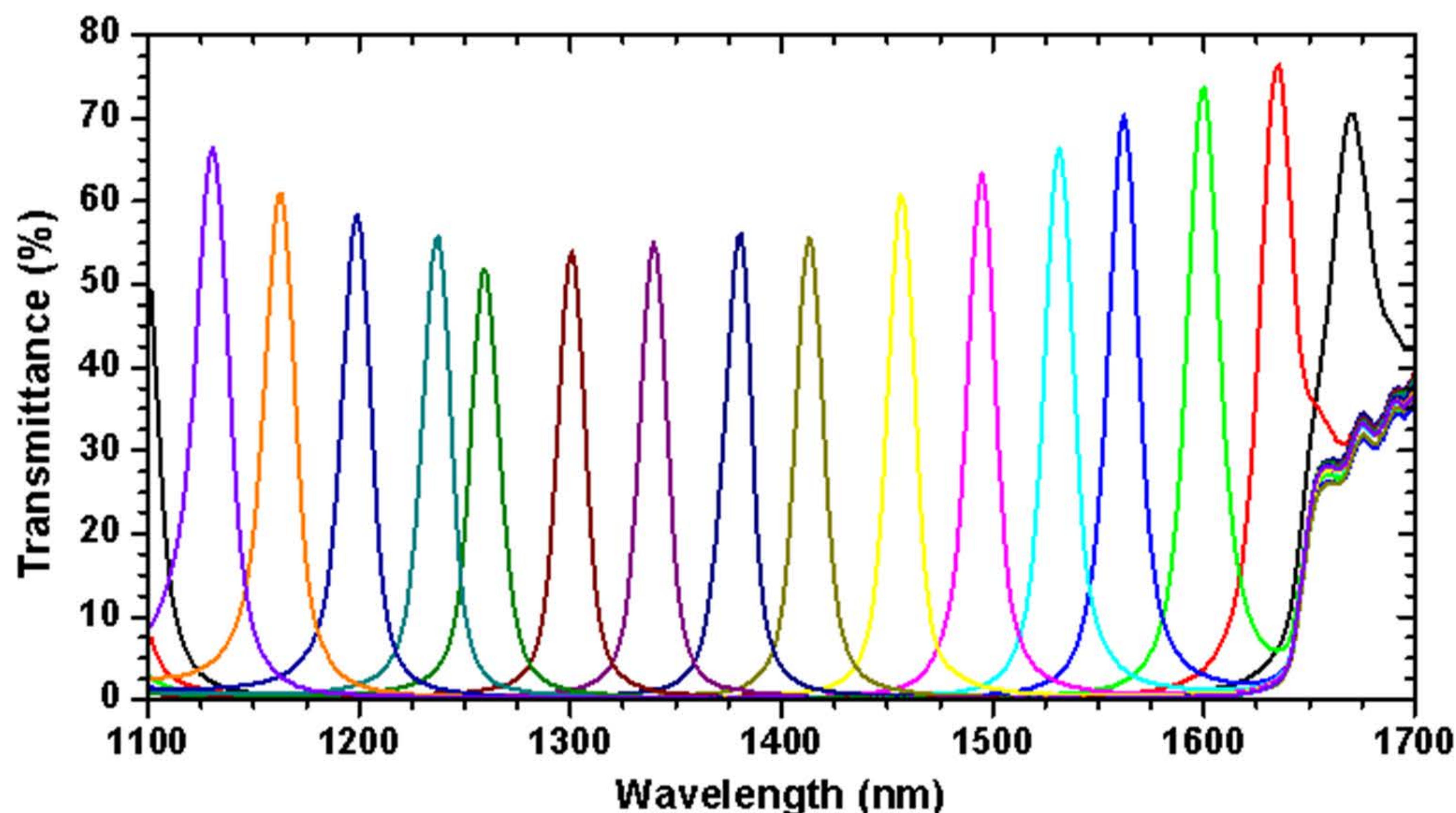
16通道1100-1700nm波段光谱曲线
