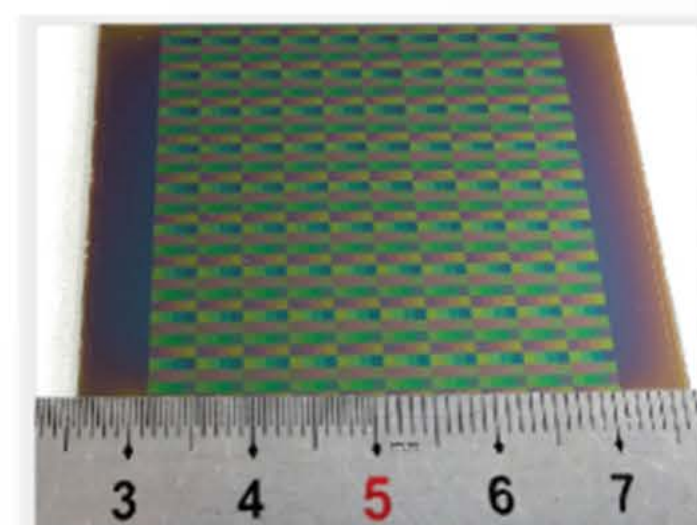
16通道滤光片实物图
